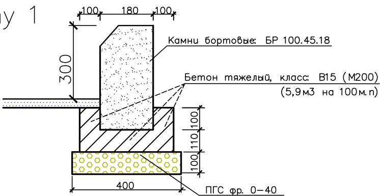
Узел бортового камня БР 100.45.18
