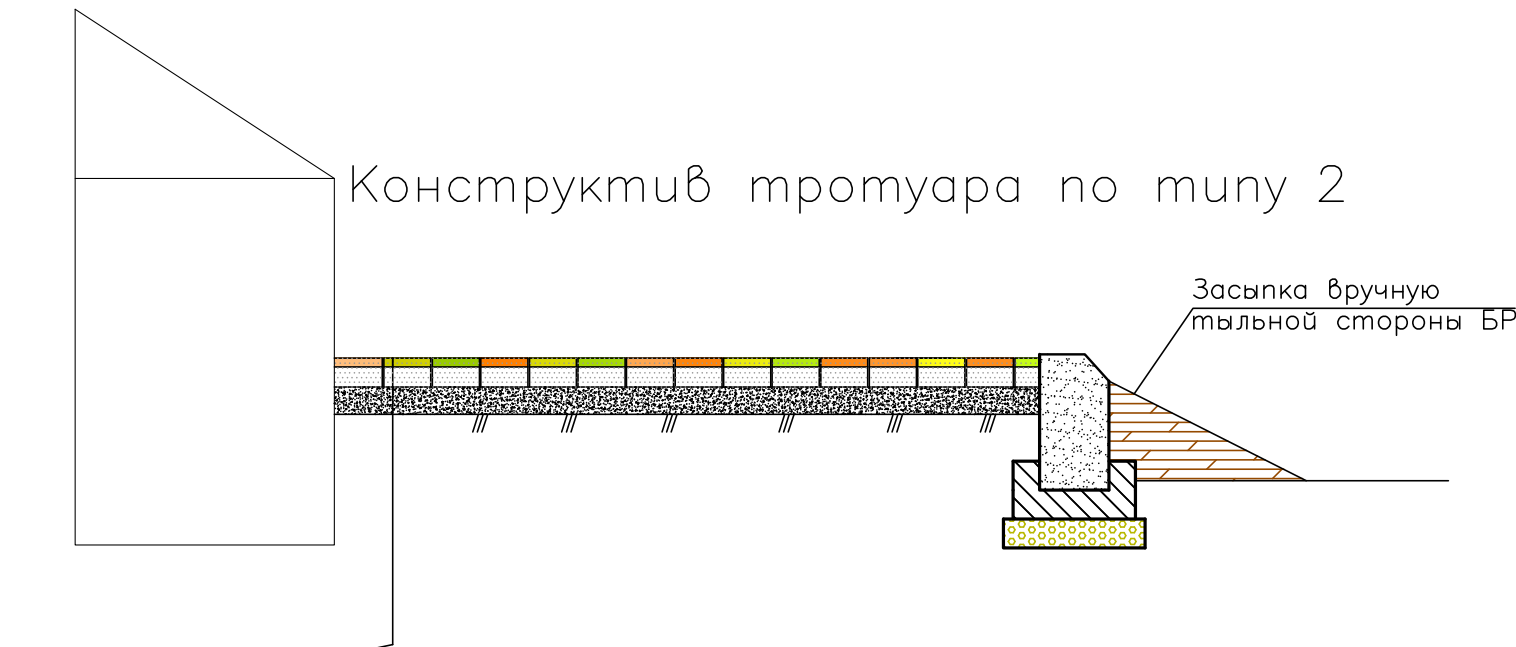
Узел бортового камня БР 100.45.18
